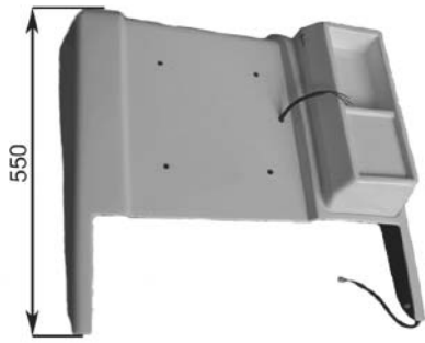
2004 Cesab Blitz-Btcbce 312-315-412-415
