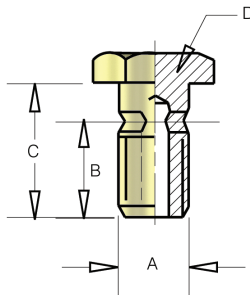
Raccordo forato senza battuta Pierced connection without rim
