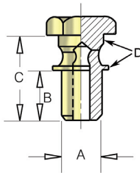
Raccordo forato con battuta Pierced connection with rim
